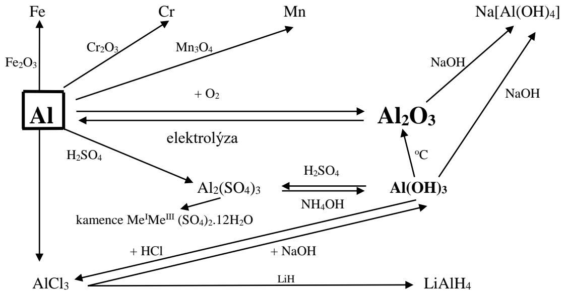
Reakce hliníku a jeho sloučenin
