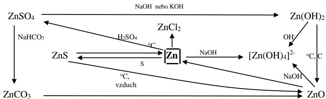
Reakce zinku a jeho sloučenin.
