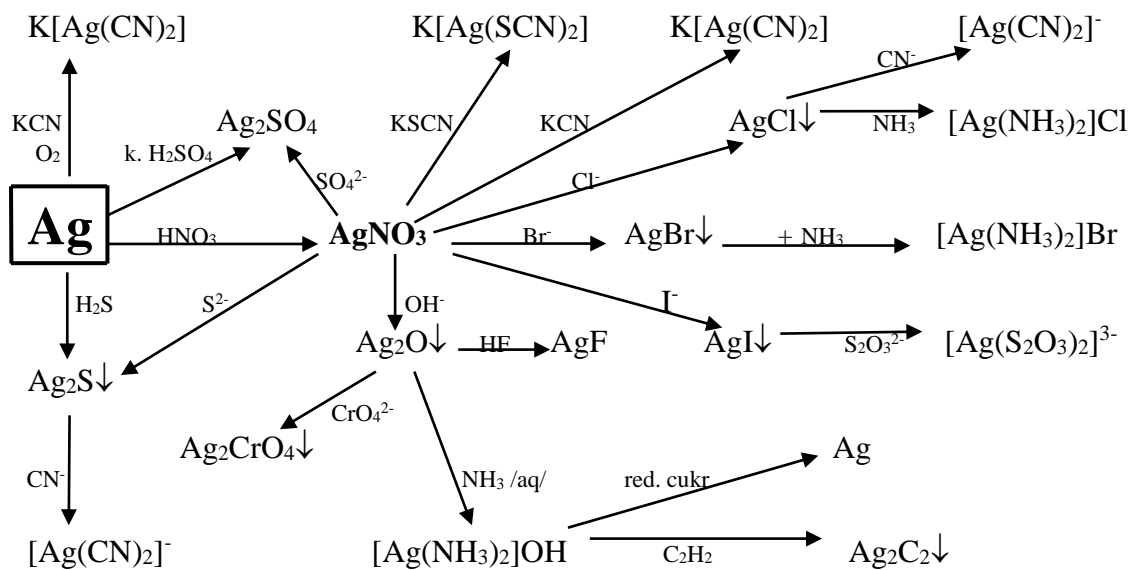
Reakce stříbra a jeho sloučenin
