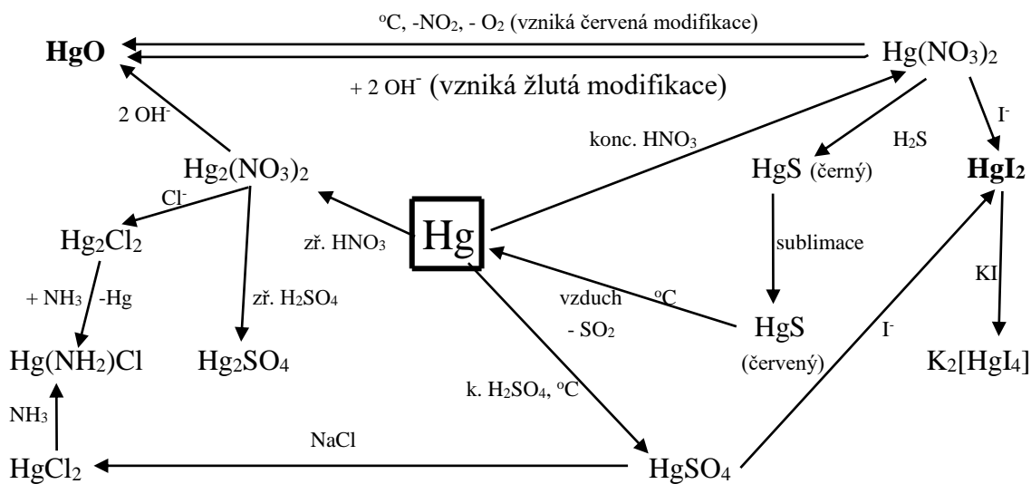
Reakce rtuti a jejich sloučenin.
