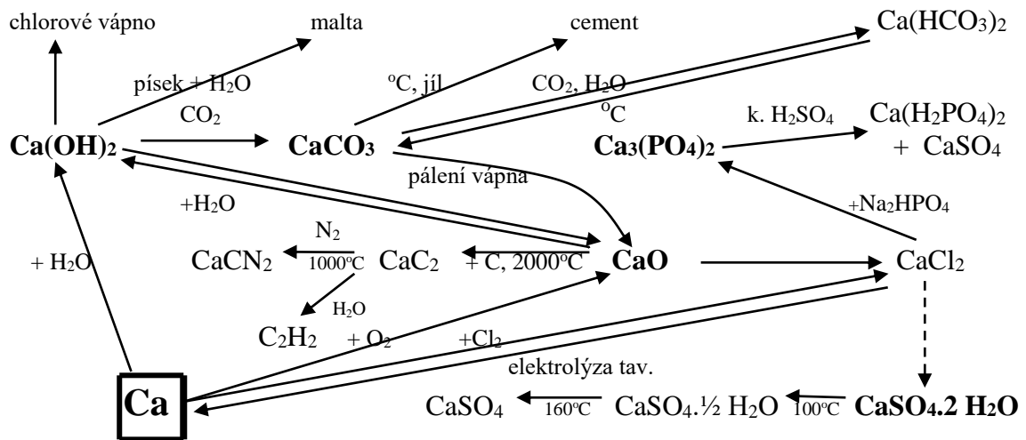
Reakce vápníku a jeho sloučenin
