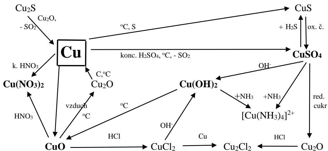
Reakce mědi a jejich sloučenin
