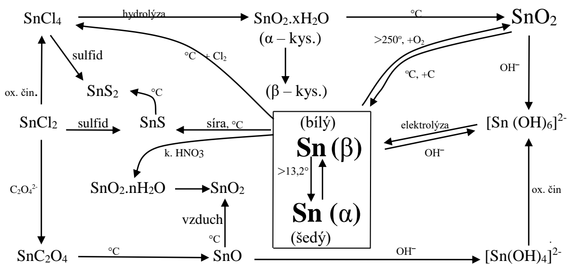
Reakce cínu a jeho sloučenin.
